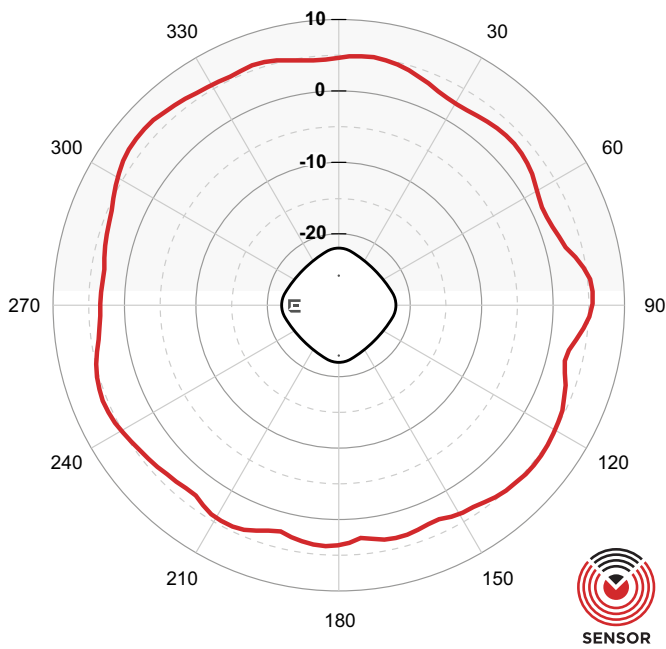
AZYMUT 5 GHz SENSOR
