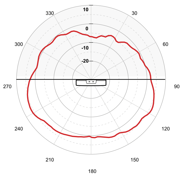
ELEWACJA 5 GHz
