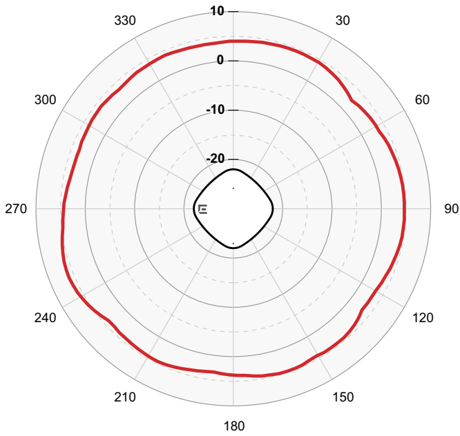
AZYMUT 2.4 GHz
