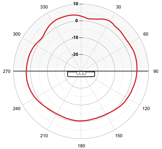
ELEWACJA 2.4 GHz
