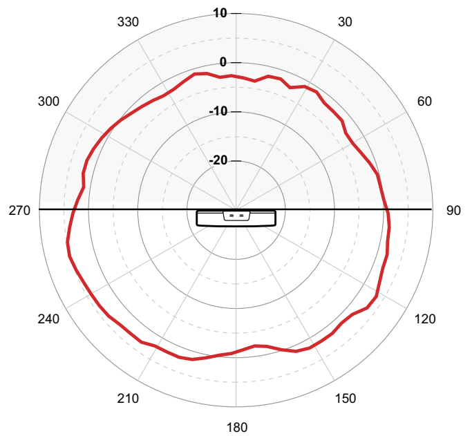
ELEWACJA 6 GHz
