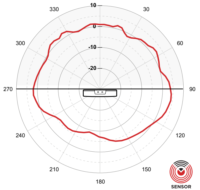
ELEWACJA 6 GHz SENSOR
