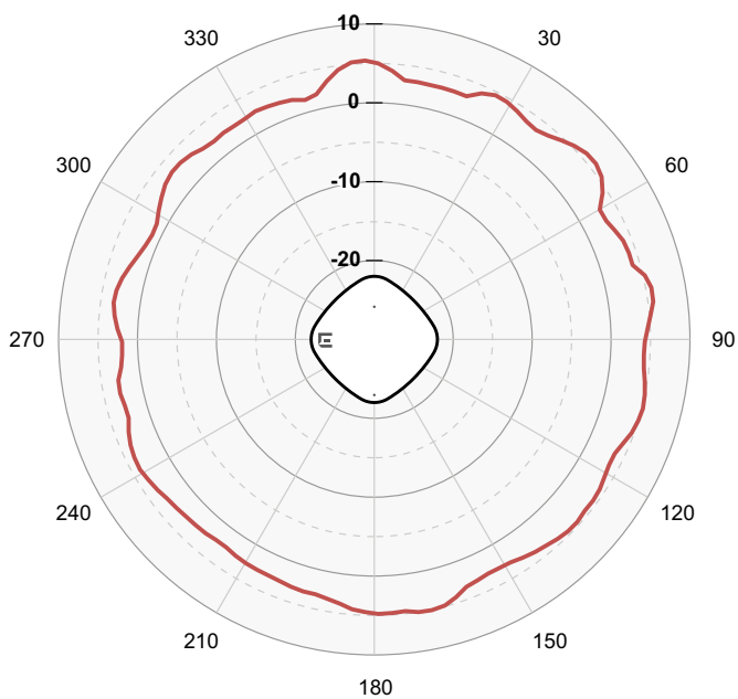
AZYMUT 5 GHz
